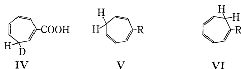
IV a: R=COOH b: R=CN c: R=Ph V a: R=COOH b: R=CN c: R=Ph VI a: R=COOH b: R=Ph
