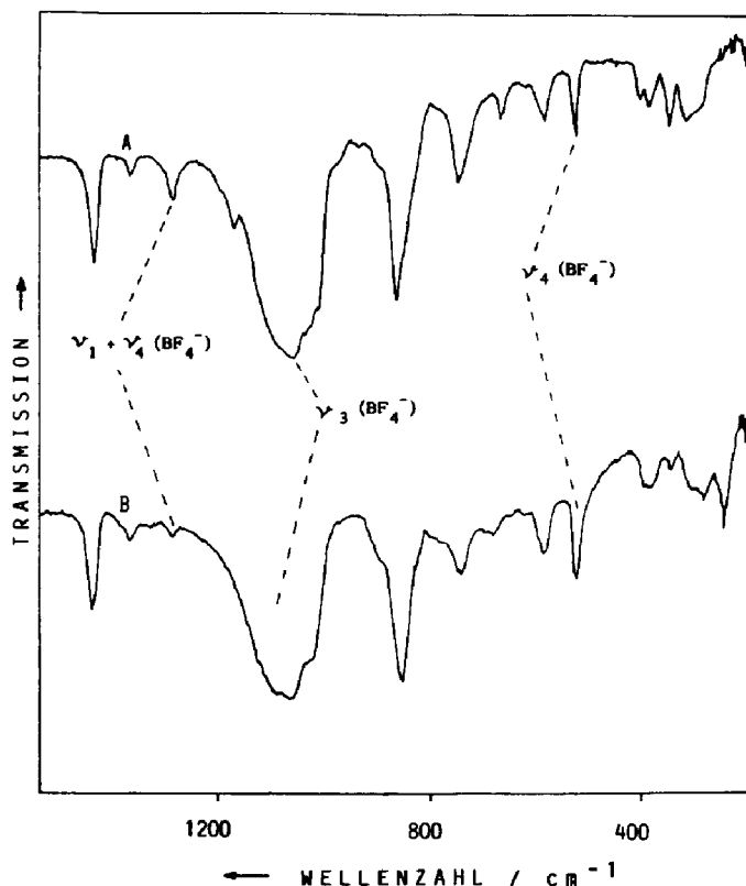
Fig. 2. IR-Spektrum von III (CsI-Preßling), dargestellt gemäß Gleichung 2 (A) und Gleichung 11 (B).
