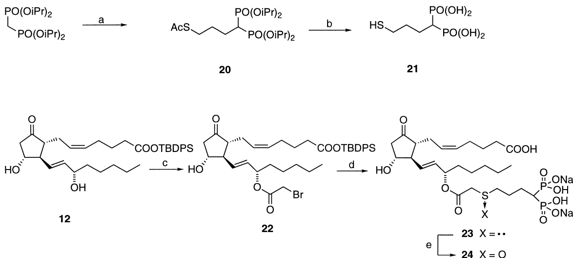
Scheme 5. Reagents: (a) NaH, DMF, AcS(CH 2 ) 3 I ( 19 ); (b) HCl, reflux; (c) BrCH 2 COBr, THF, pyr, −25°C; (d) 1) 21 , Et 3 N, dioxane, water. 2) DOWEX (Na + ); (e) CH 3 COOOH.
