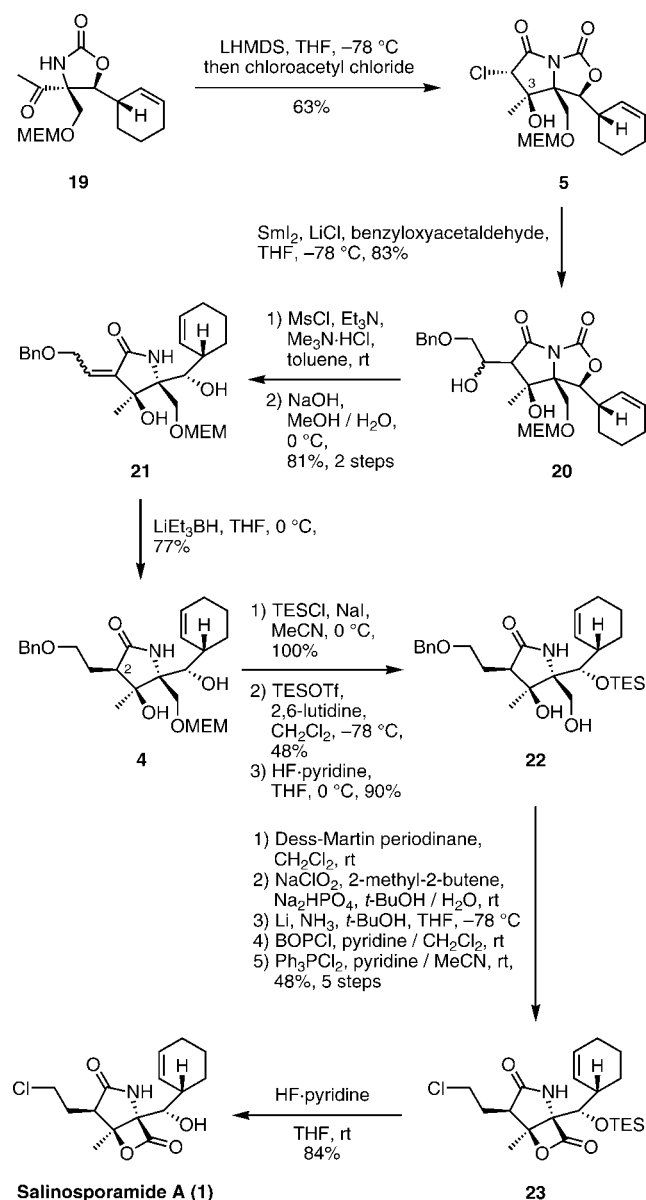
Salinosporamide A ( 1 )
