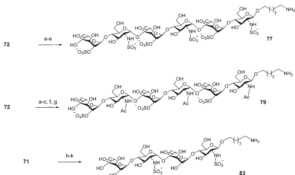
Scheme 10. Preparation of oligosaccharides 77 , 79 and 83 . a) LiOH, H 2 O 2 ; KOH, MeOH, 86 % ( 73 ); b) SO 3 ·Et 3 N, DMF, 55 °C, 86 % ( 74 ); c) PMe 3 , THF, NaOH, 69 % ( 75 ); d) SO 3 ·Py, Py, TEA, 92 % ( 76 ); e) H 2 , Pd/C, 95 % ( 77 ); f) Ac 2 O, TEA, MeOH, 94 % ( 78 ); g) H 2 , Pd/C, 90 % ( 79 ); h) LiOH, H 2 O 2 ; KOH, MeOH, 82 % ( 80 ); i) PMe 3 , THF, NaOH, quant. ( 81 ); j) SO 3 ·Py, TEA, MeOH, NaOH, 82 % ( 82 ); k) H 2 , Pd/C, 85 % ( 83 ).
