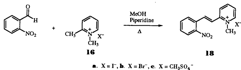
Scheme VI
