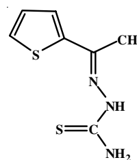
Fig. 2. Structure of ATT ligand
