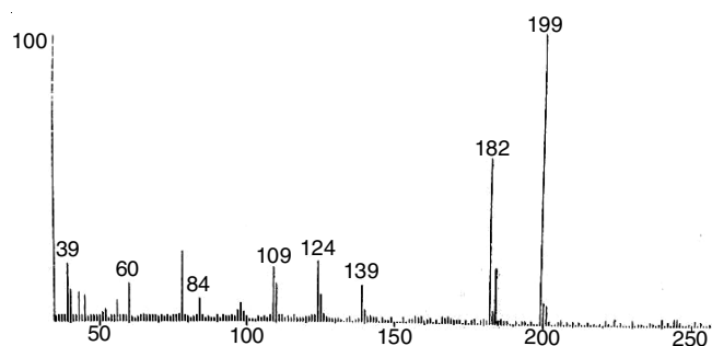
Fig. 1. Mass spectrum of ATT ligand
