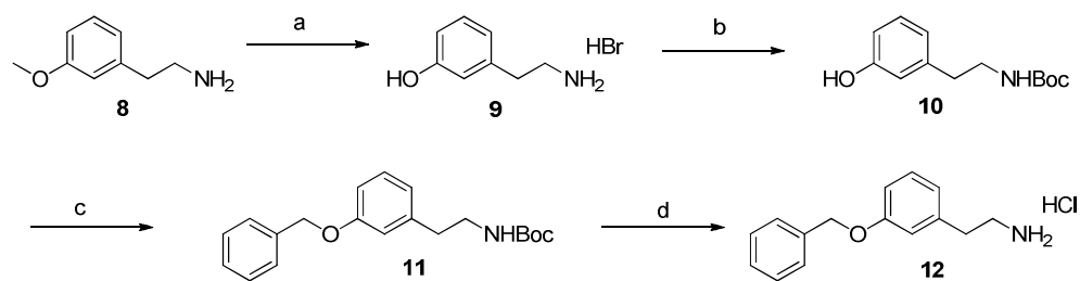
Scheme 2. a) HBr, AcOH, reflux, 4h, quant.; b) Et 3 N, Boc 2 O, DMF/dioxane, 18 h, 84%; c) Cs 2 CO 3 , BnBr, MeCN, 24 h, 75%; d) HCl, Et 2 O.
