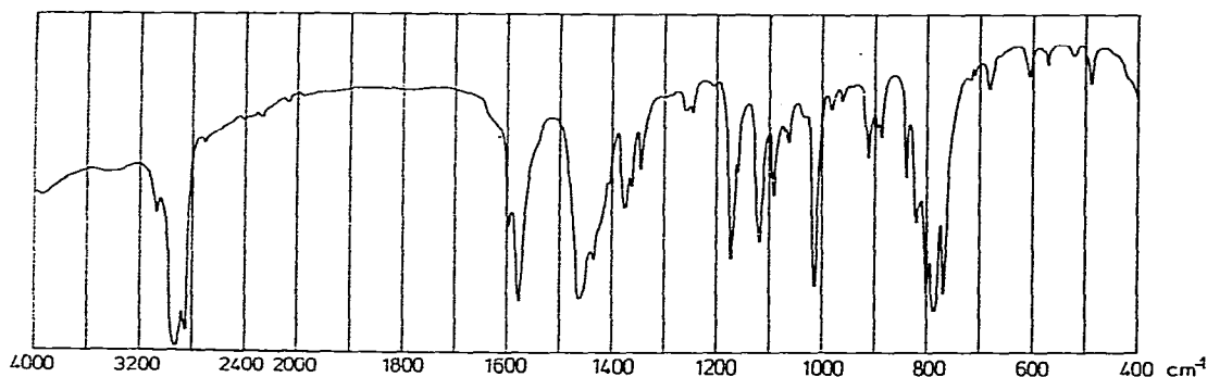
Fig. 2. IR spectrum of \text{Cp}_2\text{TiC(CH}_3\text{)=N-2,6-(CH}_3)_2\text{C}_6\text{H}_3 (KBr, Nujol).
