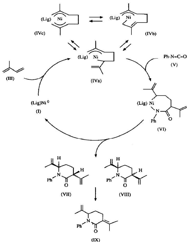
Schema 1. Katalysezyklus zur Herstellung von VII, VIII und IX am (Lig)Ni 0 -System, Lig = P(O-cyclo-C 6 H 11 ) 3 .
