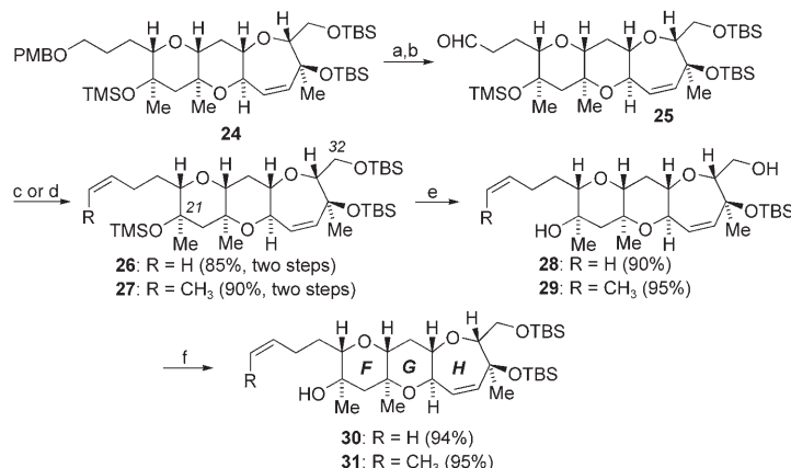
Scheme 5. a) DDQ, \text{H}_2\text{O} , \text{CH}_2\text{Cl}_2 (98%); b) TPAP, NMO; c) \text{PPh}_3\text{PCH}_2 ; d) \text{Ph}_3\text{PCHCH}_3 ; e) CSA, MeOH; f) TBSCl, \text{NEt}_3 , DMAP, \text{CH}_2\text{Cl}_2 ; DDQ: 2,3-dichloro-5,6-dicyano-1,4-benzoquinone.
