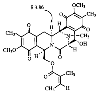
renieramycin C
