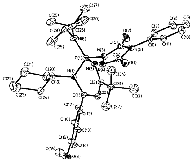
Fig. 2. Crystal structure of 12 . Selected bond lengths (pm) and bond angles ( ^{\circ} ): \text{P1--N1} 164.4(5) , \text{P1--N2} 162.5(5) , \text{N1--C1} 141.3(9) , \text{C1--C2} 135.2(10) , \text{C2--C3} 144.0(9) , \text{N2--C3} 132.4(8) , \text{P1--N6} 161.1(6) , \text{P1--N3} 165.6(6) , \text{N4--C4} 132.3(9) , \text{N3--C5} 136.8(9) , \text{C4--O1} 124.4(9) , \text{C5--O2} 122.0(9) , \text{N5--C4} 145.1(9) , \text{N5--C5} 137.7(9) , \text{N3--N4} 145.1(8) , \text{N6--P1--N2} 110.8(3) , \text{N6--P1--N1} 114.8(3) , \text{N2--P1--N1} 107.2(3) , \text{N6--P1--N3} 109.9(3) , \text{N2--P1--N3} 110.6(3) , \text{N1--P1--N3} 103.3(3) , \text{C1--N1--P1} 112.8(5) , \text{C1--N1--C19} 122.8(6) , \text{C19--N1--P1} 122.4(5) , \text{C25--N6--C28} 116.5(6) , \text{C25--N6--P1} 117.6(5) , \text{C28--N6--P1} 125.4(5) , \text{N4--C4--N5} 110.4(7) , \text{N3--C5--N5} 104.1(7) .
