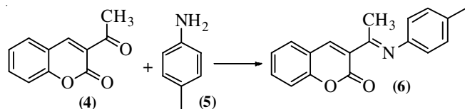
Fig. 2. Synthesis of (E)-3-(1-( p -tolylimino)ethyl)-2H-chromen-2-one
