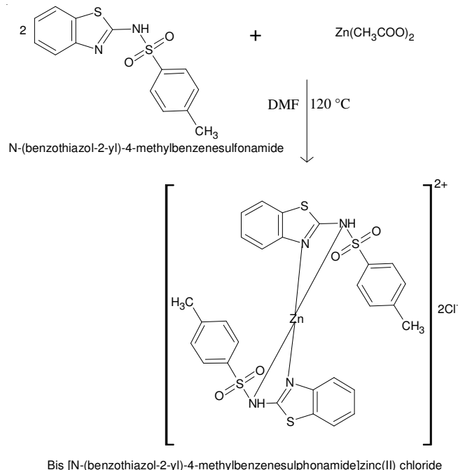
Scheme-V: Synthesis of bis -[ N -(benzothiazol-2-yl)-4-methylbenzenesulphonamide] zinc(II) chloride (Zn(II)PTS2ABT)
