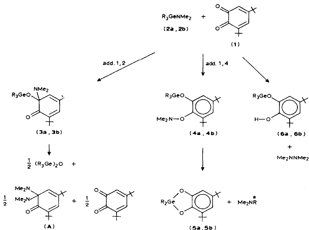
Schéma 1. a: R = C_2H_5 ; b: C_6H_5 .
