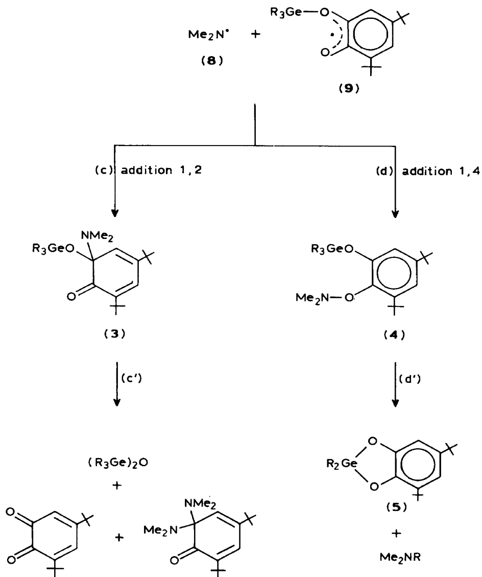
Schéma 2. Réactions dans la cage de solvant.
