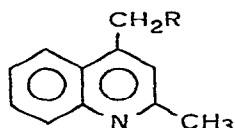
4 , R = H ; 4b , R = Li
