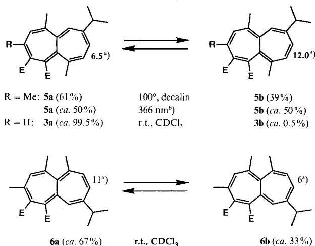
Scheme 4 a)
