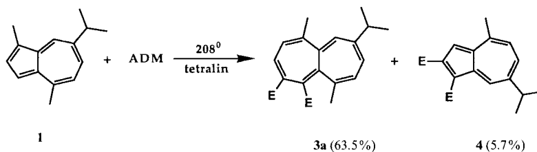
Scheme 2 a)
