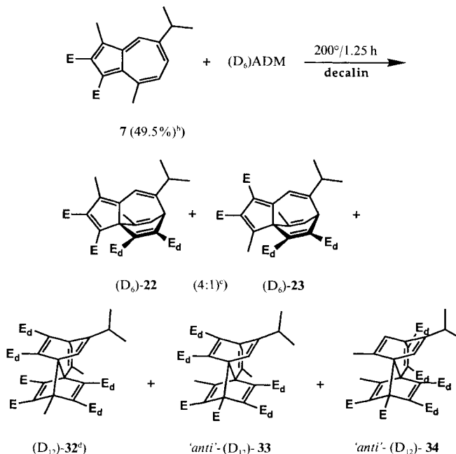
Scheme 11 a)
