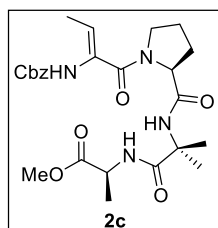
Methyl (2-((S)-1-((Z)-2-(((Benzyloxy)carbonyl)amino)but-2-enoyl)pyrrolidine-2-
