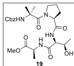
Methyl (2-(((Benzyloxy)carbonyl)amino)-2-methylpropanoyl)-L-prolyl-L-
