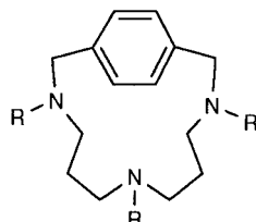
12a R = H b R = (EtO) 2 P(O)
