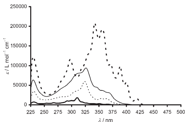
Figure 8. Electronic absorption spectra of 5 (-----), 9 (—), 11 (.....), and 31 (—).
