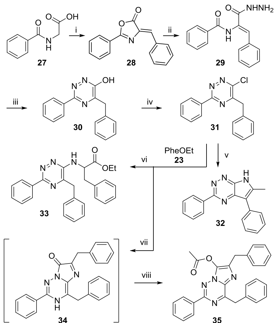
Scheme 4. i: PhCHO, AcONa, Ac 2 O, 65 - 90 °C. ii: NH 2 NH 2 , EtOH, 20 °C. iii: NaOH 1.5N, reflux. iv: POCl 3 , K 2 CO 3 , MeCN, reflux. v: Pd(OAc) 2 , BINAP, Cs 2 CO 3 , MeCN, 60 °C. vi: Pd(OAc) 2 , BINAP, Cs 2 CO 3 , toluene, 90 °C. vii: NEt 3 , NMP, 120 °C, 14 days. viii: Ac 2 O, NEt 3 , 20 °C.
