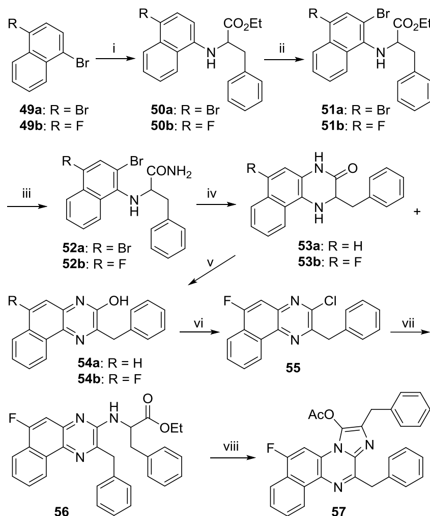
Scheme 7. i: PheOEt ( 23 ), Pd(OAc) 2 , BINAP, Cs 2 CO 3 , toluene, 100 - 105 °C. ii: NBS, CH 2 Cl 2 , 0-20 °C. iii: 7N NH 3 /MeOH, 100 °C. iv: Pd(OAc) 2 , Xantphos, Cs 2 CO 3 , THF, 120 °C. v: 35% AcOOH/AcOH, AcOEt, 20 °C. vi: PhPOCl 2 , 100 °C. vii: PheOEt ( 23 ), Pd(OAc) 2 , BINAP, Cs 2 CO 3 , MeCN, 60 °C. viii: 1) NaOH, THF, 20 °C, 2) Ac 2 O, 20 °C.
