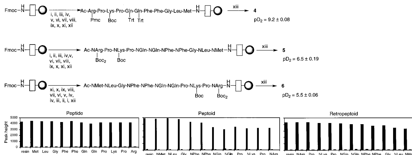
Scheme 5. Solid-phase syntheses of substance P ( 4 ), its corresponding peptoid 5 , and retropeptoid 6 , as well as the solid-phase synthesis monitoring profiles. For 4 : i) a) piperidine, b) Fmoc-Met-OH, BOP, HOBt, DiPEA; ii) a) piperidine, b) Fmoc-Leu-OH, BOP, HOBt, DiPEA; iii) a) piperidine, b) Fmoc-Gly-OH, BOP, HOBt, DiPEA; iv) a) piperidine, b) Fmoc-Phe-OH, BOP, HOBt, DiPEA; v) a) piperidine, b) Fmoc-Phe-OH, BOP, HOBt, DiPEA; vi) a) piperidine, b) Fmoc-Gln(Trt)-OH, BOP, HOBt, DiPEA; vii) a) piperidine, b) Fmoc-Gln(Trt)-OH, BOP, HOBt, DiPEA; viii) a) piperidine, b) Fmoc-Pro-OH, BOP, HOBt, DiPEA; ix) a) piperidine, b) Fmoc-Lys(Boc)-OH, BOP, HOBt, DiPEA; x) a) piperidine, b) Fmoc-Pro-OH, BOP, HOBt, DiPEA; xi) a) piperidine, b) Fmoc-Arg(Pmc)-OH, BOP, HOBt, DiPEA; xii) a) piperidine, b) Ac 2 O, DiPEA, HOBt; xiii) TFA/thioanisole/H 2 O/EDT/TIS, 86.5/5/5/2.5/1 (v/v). For 5 and 6 : i) a) piperidine, b) Fmoc-NMet-OH ( 10c ), PyBroP, DiPEA; ii) a) piperidine, b) Fmoc-NLeu-OH ( 10b ), PyBroP, DiPEA; iii) a) piperidine, b) Fmoc-Gly-OH, PyBroP, DiPEA; iv) a) piperidine, b) Fmoc-NPhe-OH ( 10a ), PyBroP, DiPEA; v) a) piperidine, b) 10a , PyBroP, DiPEA; vi) a) piperidine, b) Fmoc-NGln-OH ( 10e ), PyBroP, DiPEA; vii) a) piperidine, b) 10e , PyBroP, DiPEA; viii) a) piperidine, b) Fmoc-Pro-OH, PyBroP, DiPEA; ix) a) piperidine, b) Fmoc-NLys(Boc)-OH ( 10d ), PyBroP, DiPEA; x) a) piperidine, b) Fmoc-Pro-OH, PyBroP, DiPEA; xi) a) piperidine, b) Fmoc-NArg(Boc) 2 -OH ( 21 ), PyBroP, DiPEA; xii) a) piperidine, b) Ac 2 O, DiPEA, HOBt; xiii) TFA/thioanisole/H 2 O/EDT/TIS, 86.5/5/5/2.5/1 (v/v).
