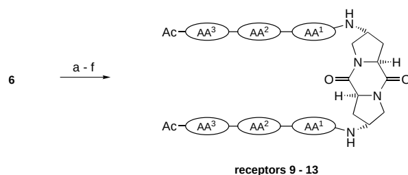
Scheme 3. Synthesis of the diketopiperazine receptors 9–13 : a) i) \text{TFA} , \text{CH}_2\text{Cl}_2 ; ii) i\text{Pr}_2\text{NEt} , 7 , \text{CH}_2\text{Cl}_2 ; b) \text{HCl} , \text{MeOH} , dioxane; c) i\text{Pr}_2\text{NEt} , N - \alpha -Fmoc-amino acid, \text{EDC} , \text{CH}_2\text{Cl}_2 ; d) TAEA, \text{CH}_2\text{Cl}_2 ; e) repetition of c) and d); f) \text{Ac}_2\text{O} , \text{NEt}_3 .
