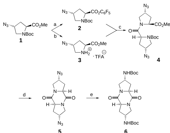
Scheme 1. Synthesis of the diketopiperazine template 6 : a) i) \text{NaOH} , \text{MeOH} , \text{THF} , \text{H}_2\text{O} ; ii) \text{C}_6\text{F}_5\text{OH} , \text{EDC} , \text{CH}_2\text{Cl}_2 , 85%; b) \text{TFA} , \text{CH}_2\text{Cl}_2 , quant.; c) i\text{Pr}_2\text{NEt} , \text{CH}_2\text{Cl}_2 , 89%; d) i) \text{TFA} , \text{CH}_2\text{Cl}_2 ; ii) i\text{Pr}_2\text{NEt} , \text{CH}_2\text{Cl}_2 , 79%; e) 10% \text{Pd/C} , \text{H}_2 , \text{MeOH} , \text{Boc}_2\text{O} , 91%.
