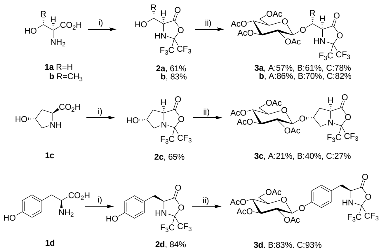
Scheme 1: i) HFA, DMSO, rt; ii) method A : Ac 4 - \alpha -D-Glc-Br, Hg(CN) 2 , CH 3 CN; method B : Ac 4 - \beta -D-Glc-OAc, BF 3 ·Et 2 O, CH 2 Cl 2 ; method C : Ac 4 - \beta -D-Glc-O-C(=NH)CCl 3 ; BF 3 ·Et 2 O, CH 2 Cl 2 .
