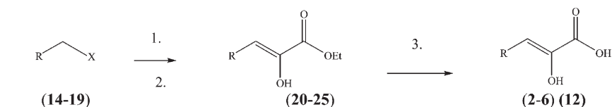
Scheme 2 1. Mg, Et 2 O, reflux, 10 min; 2. (EtOCO) 2 , Et 2 O, 0 °C, 2 h; 3. AcOH, H 2 SO 4 10%, Δ, 1 h.
