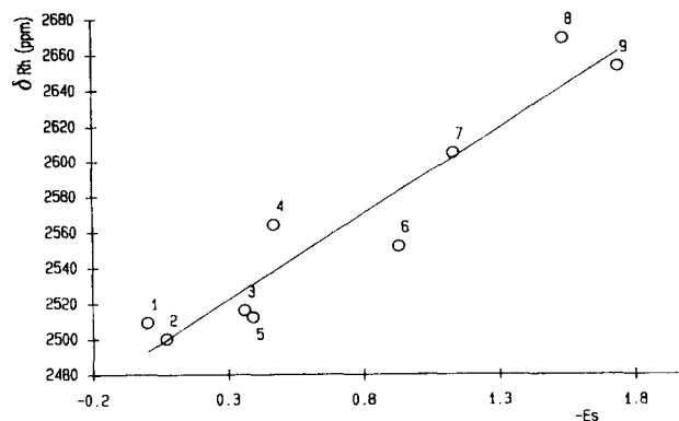
Fig. 3. ^{103}\text{Rh} chemical shifts in [\text{Rh}(\text{Hdmg})_2\text{Rpy}] vs. -Es ( R = \text{Me} (1), \text{Et} (2), ^n\text{Pr} (3), ^i\text{Pr} (4), ^n\text{Bu} (5), ^i\text{Bu} (6), ^s\text{Bu} (7), ^t\text{Bu} (8), ^{nc}\text{Pent} (9)).
