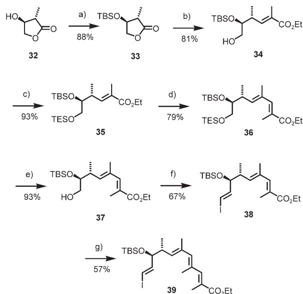
Scheme 6. a) t BuMe 2 SiOTf, 2,6-lutidine, CH 2 Cl 2 , 0 °C; b) i) DIBAH, CH 2 Cl 2 , −78 °C; ii) Ph 3 P=CCH 3 CO 2 Et, toluene, 100 °C; c) Et 3 SiCl, imidazole, CH 2 Cl 2 , 0 °C; d) i) DIBAH, toluene, −78 °C; ii) MnO 2 , CH 2 Cl 2 , 40 °C; iii) Ph 3 P=CCH 3 CO 2 Et, toluene, 100 °C; e) camphorsulfonic acid, MeOH/CH 2 Cl 2 , 0 °C; f) i) Dess–Martin periodinane, pyridine, CH 2 Cl 2 , 20 °C; ii) CrCl 3 , CHI 3 , cat. hydroquinone, THF, 1,4-dioxane, 20 °C; g) i) DIBAH, toluene, −78 °C; ii) MnO 2 , CH 2 Cl 2 , 20 °C; iii) Ph 3 P=CCH 3 CO 2 Et, toluene, 100 °C; DIBAH = diisobutylaluminium hydride.
