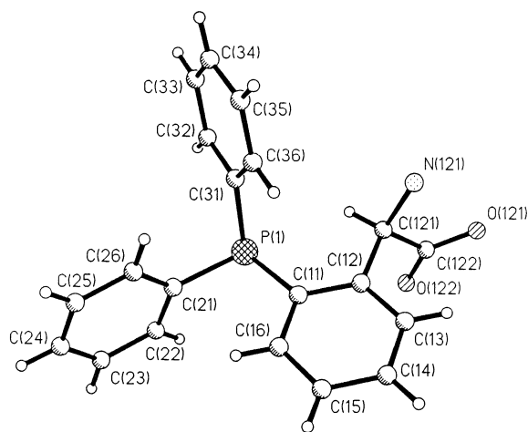
Fig. 1. Molecular structure of 3 \cdot 2\text{H}_2\text{O} . Selected bond lengths ( \text{\AA} ) and angles ( ^\circ ): \text{P}(1)\text{--C}(11) 1.849(4), \text{P}(1)\text{--C}(21) 1.839(4), \text{P}(1)\text{--C}(31) 1.848(4), \text{C}(122)\text{--O}(121) 1.249(4), \text{C}(122)\text{--O}(122) 1.247(4), \text{C}(122)\text{--C}(121) 1.545(5), \text{C}(121)\text{--N}(121) 1.504(4); \text{C}(21)\text{--P}(1)\text{--C}(31) 100.6(2), \text{C}(21)\text{--P}(1)\text{--C}(11) 101.6(2), \text{C}(11)\text{--P}(1)\text{--C}(31) 104.4(2), \text{O}(121)\text{--C}(122)\text{--O}(122) 127.7(5), \text{N}(121)\text{--C}(121)\text{--C}(122) 108.8(3), \text{O}(122)\text{--C}(122)\text{--C}(121) 115.1(4), \text{O}(121)\text{--C}(122)\text{--C}(121) 117.2(4).
