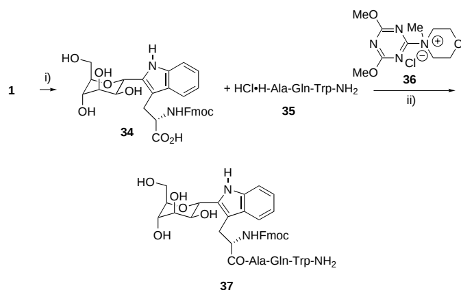
Scheme 12. i) Fmoc-OSu, \text{NaHCO}_3 , DME, \text{H}_2\text{O} (67 %); ii) 35 , 36 , MeOH (94 %).
