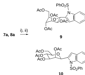
Scheme 2. i) H 2 , 20% Pd(OH) 2 /C; ii) Ac 2 O, pyridine, 9 (50%), 10 (45%).
