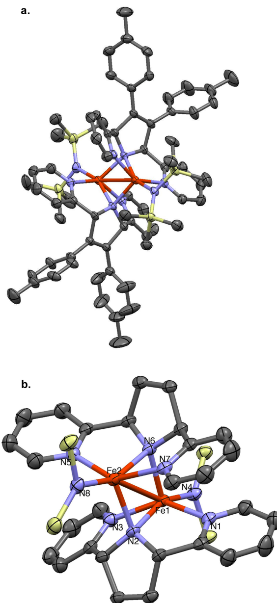
Figure 8. Molecular and truncated views of [\{2,5\text{-di}(\text{pyrindin-2-yl})\text{-3,4-di-}(p\text{-tolyl-2,5-dihydropyrrol-1-ide})\}\text{FeN}(\text{SiMe}_3)_2\}_2 ( 11 ). Selected interatomic distances ( \text{\AA} ) and angles ( ^\circ ): \text{Fe1}-\text{Fe2} , 3.054 ; \text{Fe1}-\text{N1} , 2.1411(15) ; \text{Fe1}-\text{N2} , 2.1610(15) ; \text{Fe1}-\text{N3} , 2.1632(15) ; \text{Fe1}-\text{N4} , 2.0560(15) ; \text{Fe1}-\text{N6} , 2.0966(14) ; \text{Fe2}-\text{N2} , 2.1167(14) ; \text{Fe2}-\text{N5} , 2.1775(15) ; \text{Fe2}-\text{N6} , 2.1638(15) ; \text{Fe2}-\text{N7} , 2.1500(15) ; \text{Fe2}-\text{N8} , 2.0646(15) ; \text{Fe1}-\text{N2}-\text{Fe2} , 91.10(5) ; \text{Fe1}-\text{N6}-\text{Fe2} , 91.57(5) ; \text{N1}-\text{Fe1}-\text{N2} , 78.27(6) ; \text{N1}-\text{Fe1}-\text{N3} , 143.98(6) ; \text{N1}-\text{Fe1}-\text{N4} , 96.20(6) ; \text{N2}-\text{Fe1}-\text{Fe3} , 76.49(6) ; \text{N2}-\text{Fe1}-\text{N4} , 156.89(6) ; \text{N3}-\text{Fe1}-\text{N4} , 97.02(6) ; \text{N6}-\text{Fe1}-\text{N1} , 98.10(5) ; \text{N6}-\text{Fe1}-\text{N2} , 88.57(5) ; \text{N6}-\text{Fe1}-\text{N3} , 106.48(6) ; \text{N6}-\text{Fe1}-\text{N4} , 114.51(6) ; \text{N5}-\text{Fe2}-\text{N6} , 76.43(6) ; \text{N5}-\text{Fe2}-\text{N7} , 144.10(6) ; \text{N5}-\text{Fe2}-\text{N8} , 97.02(6) ; \text{N6}-\text{Fe2}-\text{N7} , 77.88(5) ; \text{N6}-\text{Fe2}-\text{N8} , 157.21(6) ; \text{N7}-\text{Fe2}-\text{N8} , 97.05(6) ; \text{N2}-\text{Fe2}-\text{N5} , 107.18(6) ; \text{N2}-\text{Fe2}-\text{N6} , 87.97(5) ; \text{N2}-\text{Fe2}-\text{N7} , 96.48(5) ; \text{N2}-\text{Fe2}-\text{N8} , 114.76(6) .
