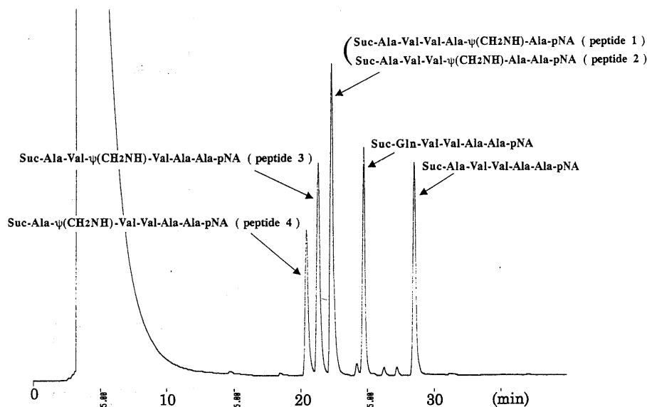
Fig. 7. HPLC Pattern of Suc-Ala-Val-Val-Ala-Ala-pNA Analogs
