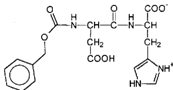
Z-Asp-His-OH (3b)
