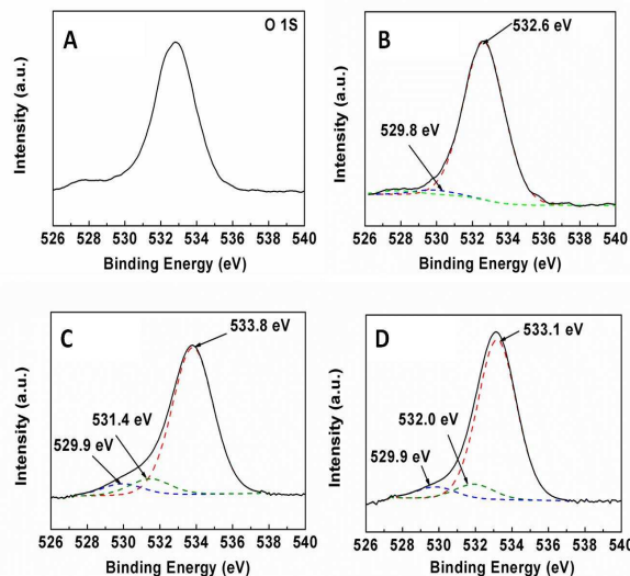
Figure 9. XPS spectra of O 1s region: (A) Si-ZSM-5; (B) 0.5 % Mn-ZSM-5; (C) 1 % Mn-ZSM-5; (D) 2 % Mn-ZSM-5.
