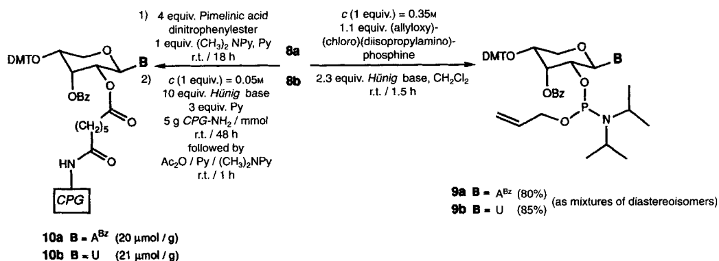
Scheme 2 (cont.)
