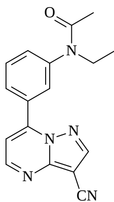
2 Zaleplon
