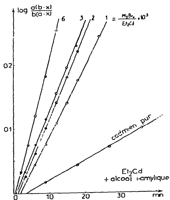
Fig. 4. Influence de la concentration en \text{MgBr}_2 sur la vitesse de réaction de \text{Et}_2\text{Cd} sur i\text{-AmOH} .
