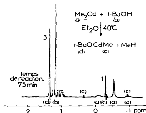
Fig. 1. Protolyse suivie en RMN (60 MHz).
