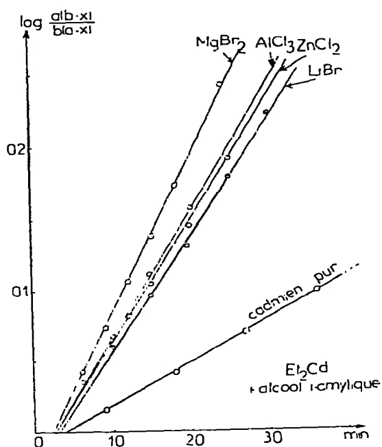
Fig. 3. Rôle des halogénures sur la vitesse de réaction de \text{Et}_2\text{Cd} sur i\text{-AmOH} .
