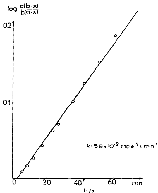
Fig. 2. Réaction de \text{Et}_2\text{Cd} sur 1-AmOH.
