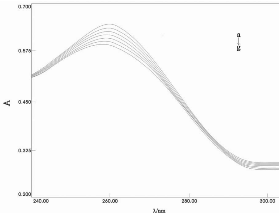
Fig. 2 UV-Vis spectra of molecular tweezers 7a ( 3 \times 10^{-4} \text{ mol L}^{-1} ) in the presence of \text{NO}_3^- . (a) 0 \text{ mol L}^{-1} ; (b) 0.024 \times 10^{-3} \text{ mol L}^{-1} ; (c) 0.024 \times 10^{-3} \text{ mol L}^{-1} ; (d) 0.048 \times 10^{-3} \text{ mol L}^{-1} ; (e) 0.048 \times 10^{-3} \text{ mol L}^{-1} ; (f) 0.072 \times 10^{-3} \text{ mol L}^{-1} ; (g) 0.072 \times 10^{-3} \text{ mol L}^{-1} with \lambda_{\text{max}} at 262.6 \text{ nm} .
