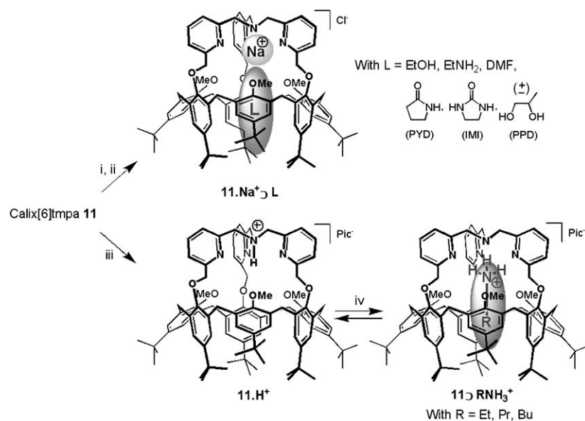
Scheme 3. i) NaCl, \text{CHCl}_3 , EtOH; ii) L (> 1 equiv), \text{CDCl}_3 ; iii) PicH (1 equiv), \text{CDCl}_3 ; iv) \text{RNH}_2 (> 1 equiv), \text{CDCl}_3 .
