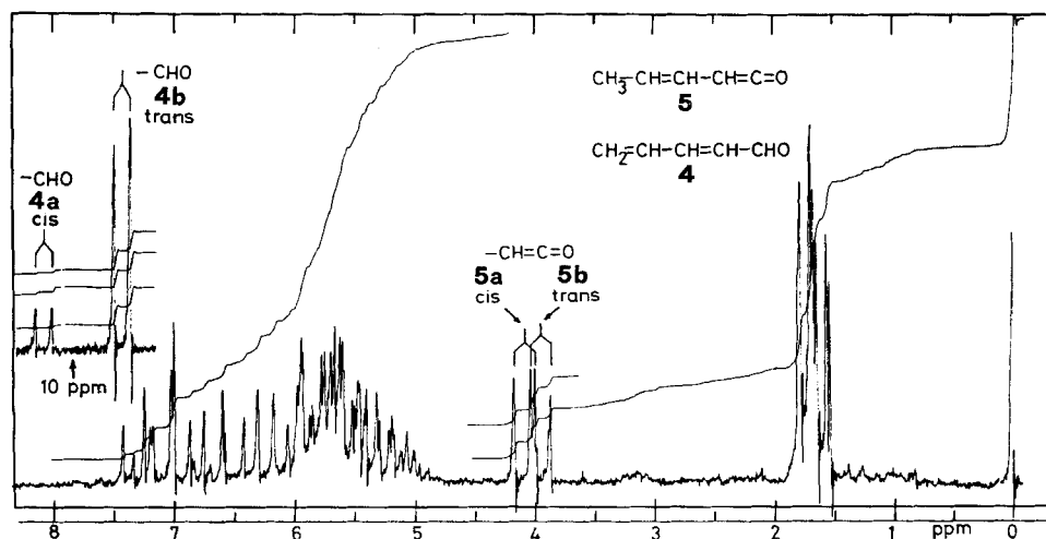
Fig. 1. NMR.-Spektrum (CS 2 , –60°) des bei 600° (0,1 s) aus (2 E )-2,4-Pentadienal ( 4b ) entstehenden Produktgemisches
