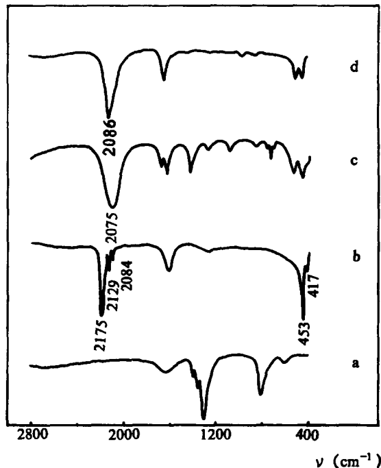
Fig. 2. Infrared spectra: (a) [\text{Co}(\text{NH}_3)_6]\text{Cl}_3 ; (b) 300°C, [\text{Co}(\text{NH}_3)_6]\text{Cl}_3 + \text{KCN} ; (c) 200°C, [\text{Co}(\text{NH}_3)_6]\text{Cl}_3 + \text{KSCN} ; (d) \text{Co}(\text{NCS})_2 .
