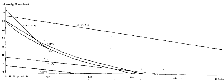
Fig. 11. \text{N}_2\text{O}_5 -Katalyse des Ozonzerfalles.
