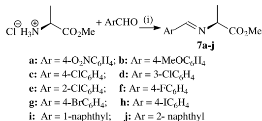
Scheme 4. Reagents: (i) Et 3 N/MgSO 4 .
