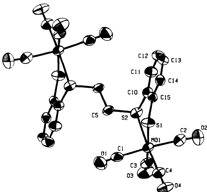
Fig. 5. Ansicht des Dianions von [\text{NMe}_4]_2[\mu\text{-dtttd}\{\text{Mo(CO)}_4\}_2] .
