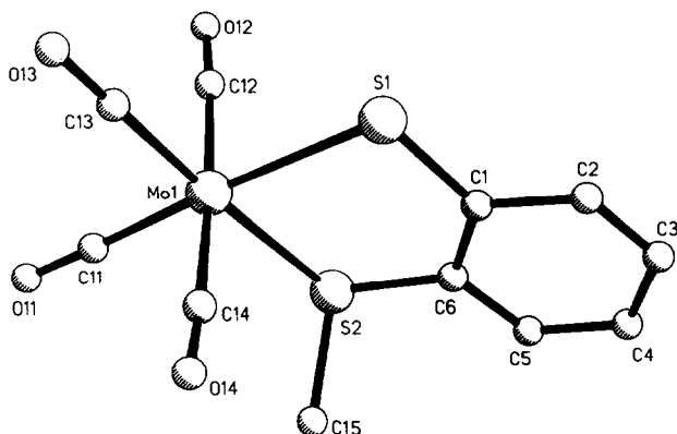
Fig. 6. Ansicht des Anions von (\text{NMe}_4)[\text{Mo}(\text{CO})_4(\text{CH}_3\text{SC}_6\text{H}_4\text{S})] (ohne H-Atome).
