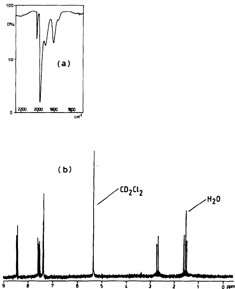
Fig. 1. (a) \nu(\text{CO}) -IR-Bereich von [\mu\text{-dtt}(\text{Mo}(\text{CO})_3)_2] \cdot 2\text{H}_2\text{O} in \text{CH}_2\text{Cl}_2 ; (b) ^1\text{H} -NMR-Spektrum (270 MHz) von [\mu\text{-dtt}(\text{Mo}(\text{CO})_3)_2] \cdot 2\text{H}_2\text{O} in \text{CH}_2\text{Cl}_2\text{-}d_2 .
