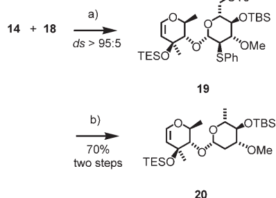
Scheme 3. a) TMSOTf, Et 2 O, -60 \rightarrow -40^\circ\text{C} , 1 h; b) i) NaI, DMF, 90^\circ\text{C} ; ii) Bu 3 SnH, AIBN, toluene, 100^\circ\text{C} .
