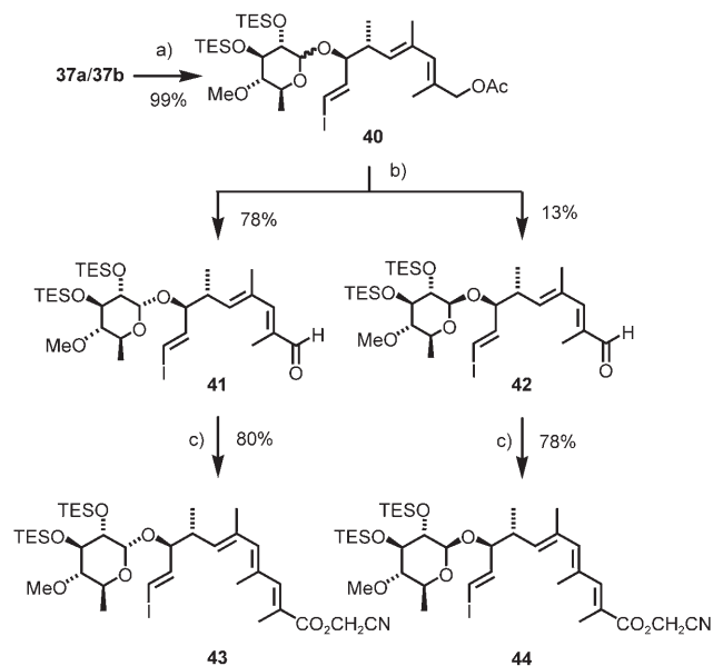
Scheme 6. a) i) TBAF, THF; ii) \text{TESCl} , imidazole; b) i) \text{LiOH} , THF/ \text{MeOH}/\text{H}_2\text{O} 2:1:1; ii) \text{MnO}_2 , \text{CH}_2\text{Cl}_2 ; c) i) (\text{EtO})_2\text{P}(\text{O})\text{CH}(\text{CH}_3)\text{CO}_2\text{H} , \text{NaH} , THF; ii) \text{ClCH}_2\text{CN} , \text{Et}_3\text{N} , \text{MeCN} , 20^{\circ}\text{C} .
