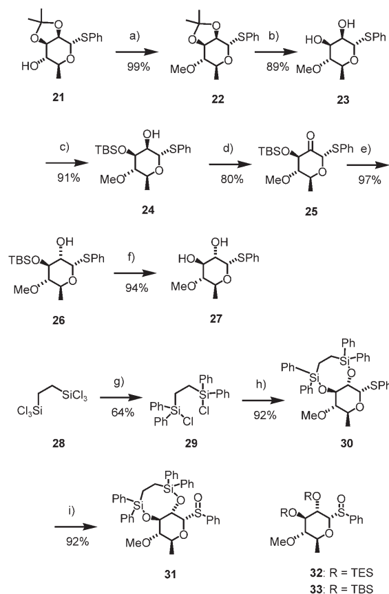
Scheme 4. a) MeI, KOH, DMF; b) p TsOH, MeOH; c) TBSCl, imidazole, DMAP; d) Dess–Martin periodinane, CH 2 Cl 2 ; e) NaBH 4 , MeOH, 0^\circ\text{C} ; f) TBAF, THF; g) PhMgBr, Et 2 O; h) 27 , imidazole, DMF; i) MCPBA, CH 2 Cl 2 , -78 \rightarrow -20^\circ\text{C} .
