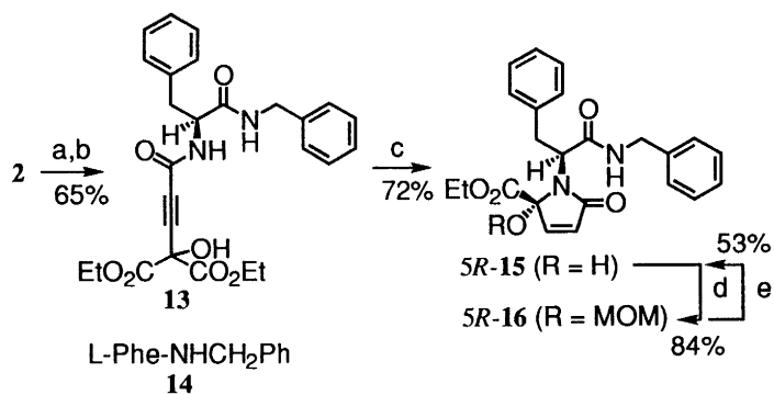
Scheme 4. (a) IBCF/MM/THF/-18°C; (b) 14/THF/-18°C→rt; (c) 1N KOH/EtOH/0°C; (d) MOMCl/DIEA/CH 2 Cl 2 /0°C→rt; (e) 4N HCl/dioxane/0°C
