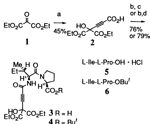
Scheme 1. (a) \text{Li}-\text{C}\equiv\text{C}-\text{Li}/\text{THF}/-78^\circ\text{C}\rightarrow\text{rt} ; (b) \text{IBCF}/\text{NMM}/\text{THF}/-16\text{--}18^\circ\text{C} ; (c) 5/\text{NMM}/\text{THF}-\text{DMF}/-18^\circ\text{C}\rightarrow\text{rt} ; (d) 6/\text{THF}/-16^\circ\text{C}\rightarrow\text{rt}
