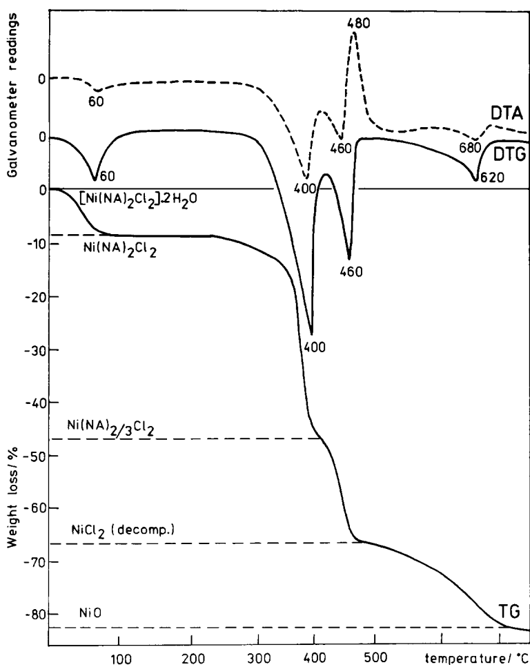
Fig. 1. Thermal curves of \text{Ni(NA)}_2\text{Cl}_2 \cdot 2\text{H}_2\text{O} .
