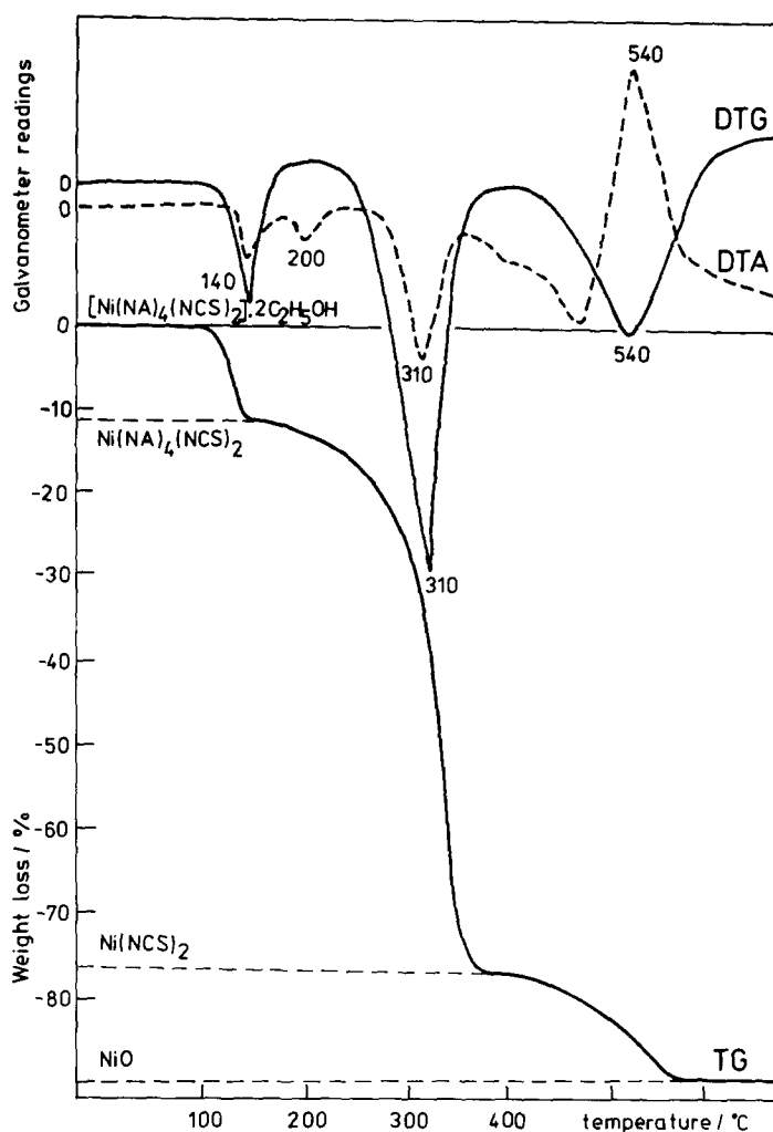
Fig. 4. Thermal curves of \text{Ni(NA)}_4(\text{NCS})_2 \cdot 2\text{C}_2\text{H}_5\text{OH} .
