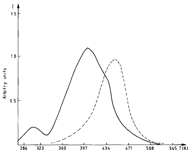
Fig. 1. Ion current curves for \text{H}_2\text{O}^+ (—) and \text{CO}_2^+ (---).
