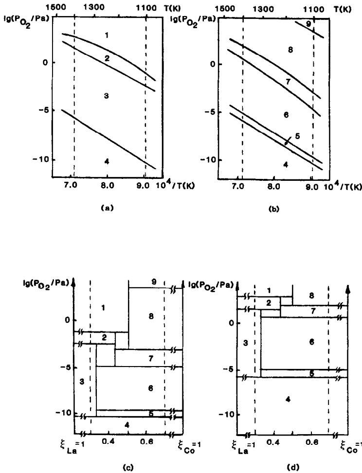
FIG. 6. Special cross section of La-Co-O system phase diagram isoconcentrational (a) for \xi_{Co} = 0.3 ; (b) for \xi_{Co} = 0.7 and isothermal (c) at 1100 K, (d) at 1400 K). Two-phase regions: 1, La_2O_3 , LaCoO_3 ; 2, La_3Co_3O_{10} , La_2O_3 ; 3, La_2CoO_4 , La_2O_4 , La_2O_3 ; 4, La_2O_3 , Co; 5, La_2CoO_4 , Co; 6, La_2CoO_4 , CoO; 7, La_4Co_3O_{10} , CoO; 8, LaCoO_3 , CoO; 9, LaCoO_3 , Co_3O_4 .
