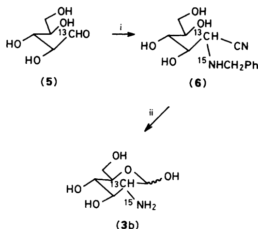
Scheme 1. Reagents: i, \text{HCN}-\text{PhCH}_2^{15}\text{NH}_2-\text{EtOH} ; ii, \text{H}_2-\text{Pd}-\text{BaSO}_4-0.5\text{M HCl}
